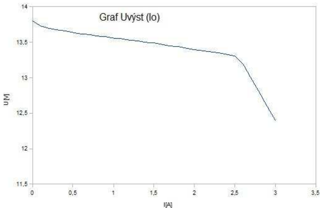
Obr. 3. Uvyst=f(Io)
