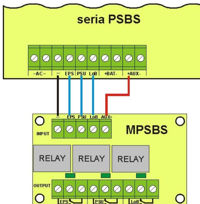
Obr. 5. Schéma zapojení modulu MPSBS.
