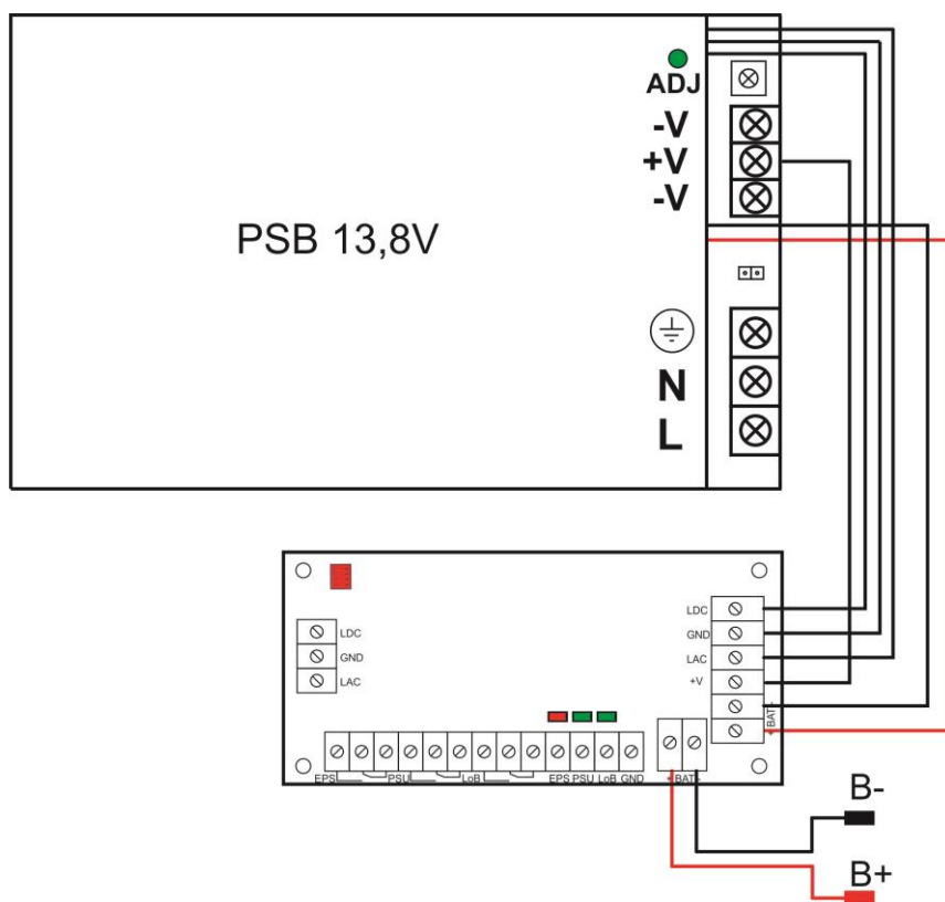
Obr.2 Schéma připojení modulu k napájecímu zdroji PSB.
