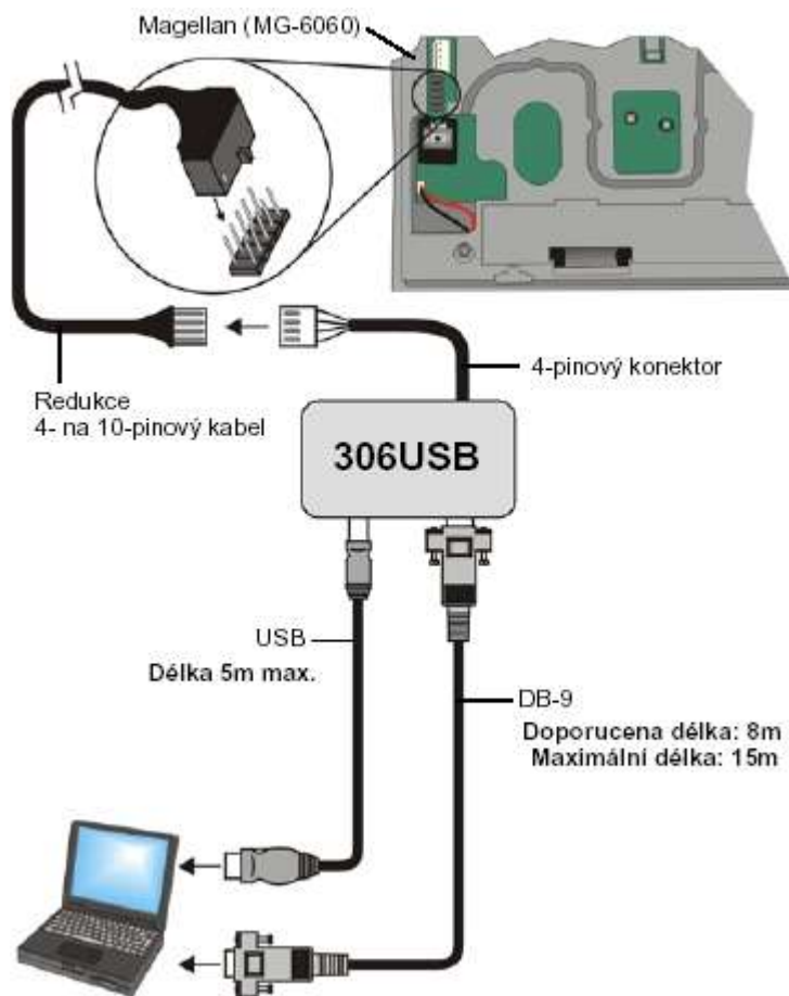
Obrázek 2 : Připojení převodníku 306USB k Magellanu
