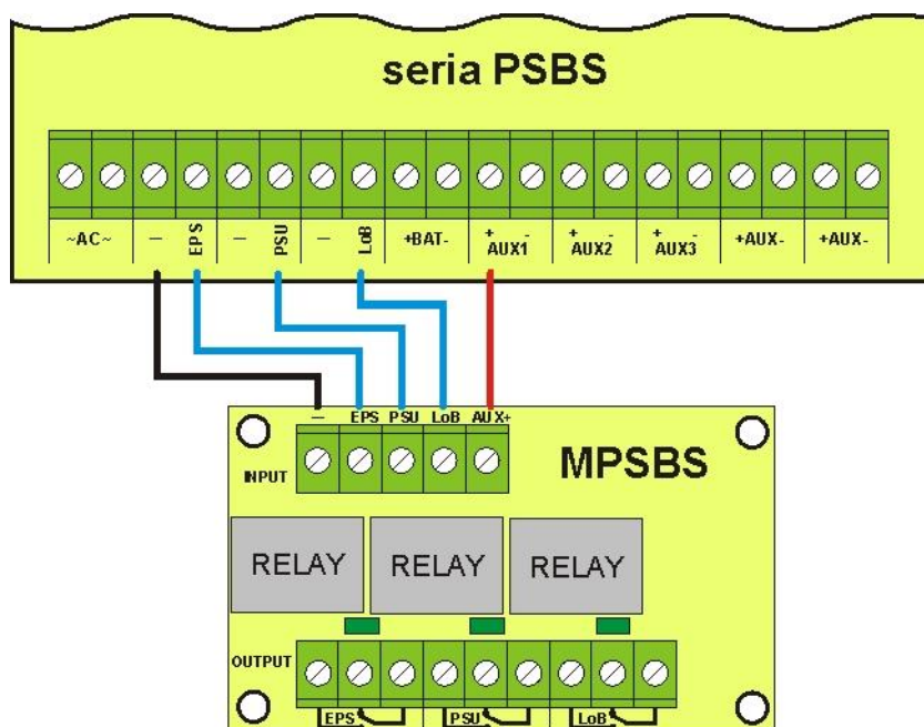
Obr. 6. Schéma zapojení modulu MPSBS.
