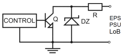
Obr. 5. Elektrické schéma technické výstupů OC.
