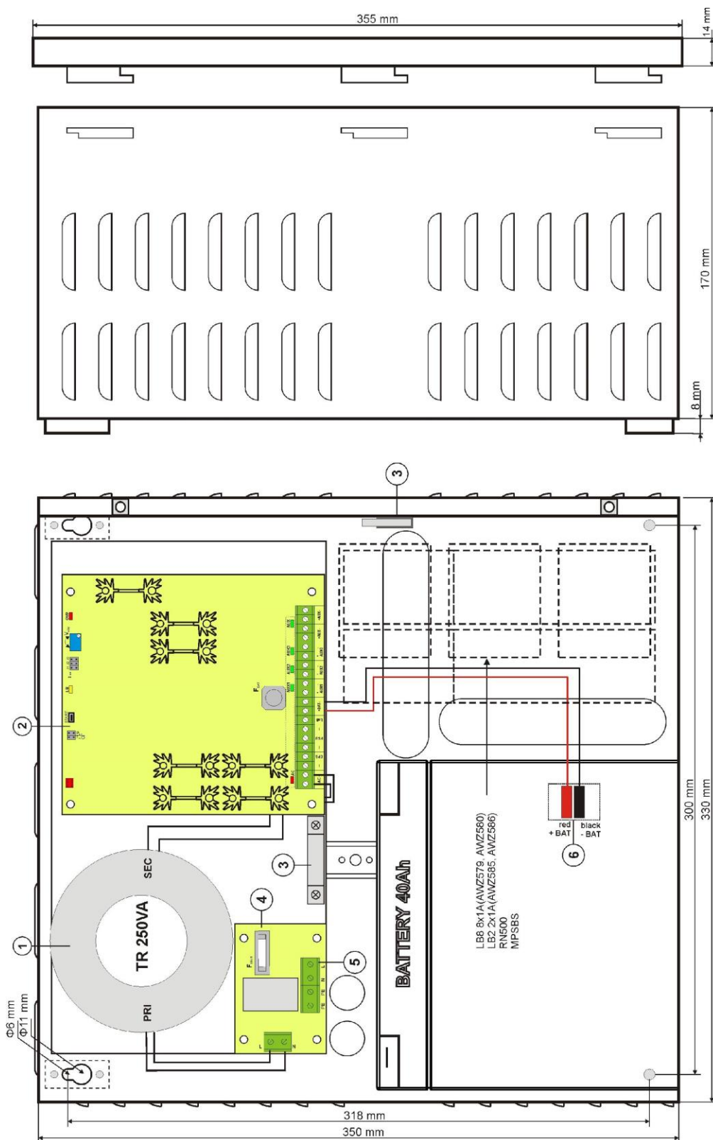
Obr.3. Náhled napájecího zdroje.
