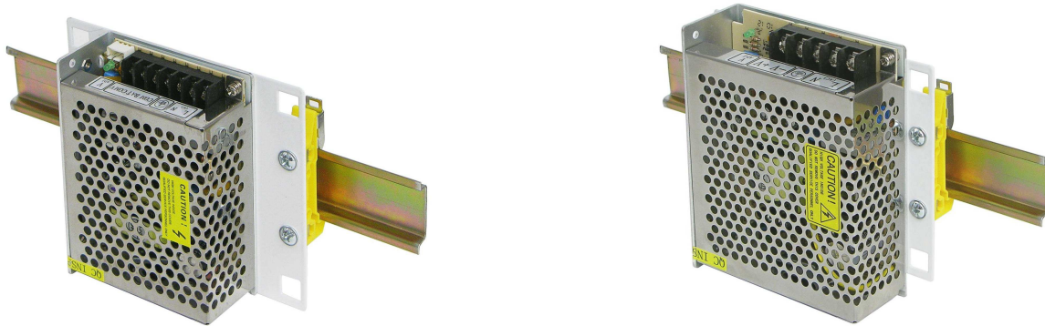
Rys. 2. Przykład montażu zasilaczy: PSB201202 i PS401203.
